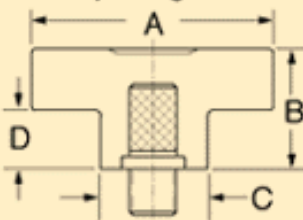
Projecting Stud
